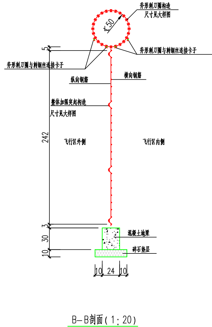
B—B剖面（1：20）
