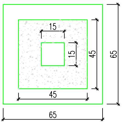
D—D剖面（1：10）
