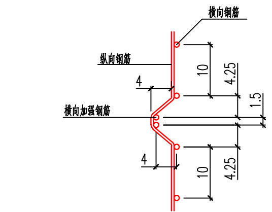
整体加强突起构造尺寸大样图（1：5）
