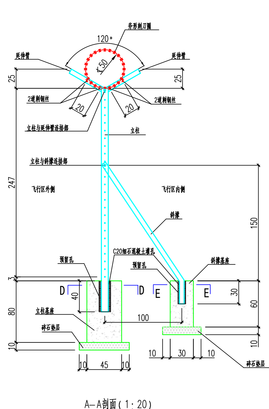
A—A剖面（1：20）
