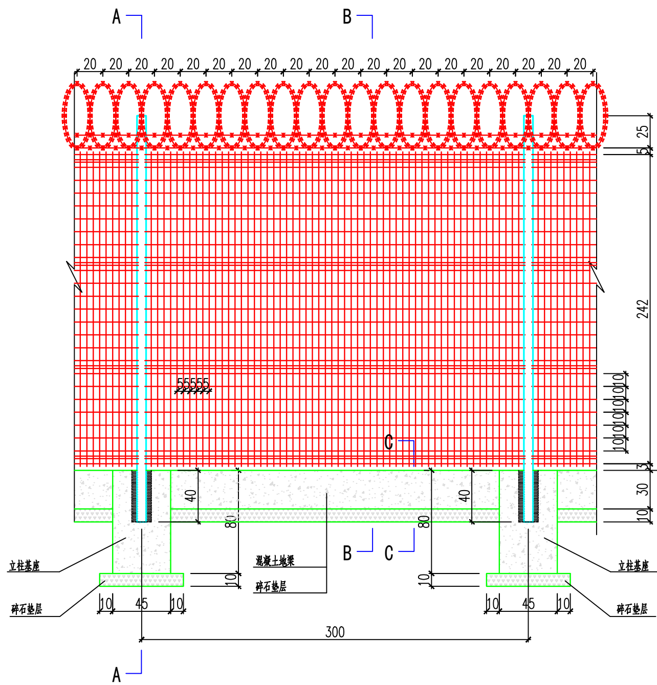
钢筋网围界立面图（外侧）（1：20）
