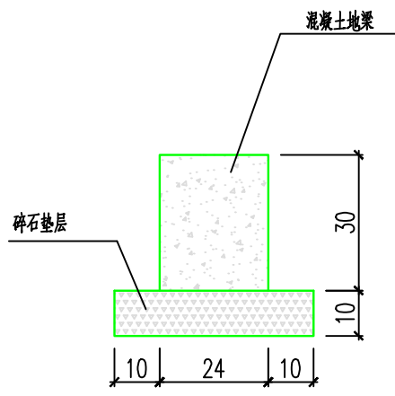
C—C剖面（1：10）
