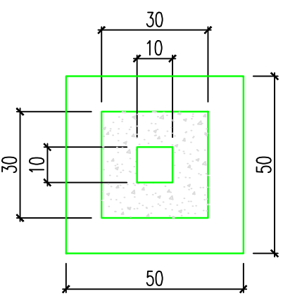
E—E剖面（1：10）
