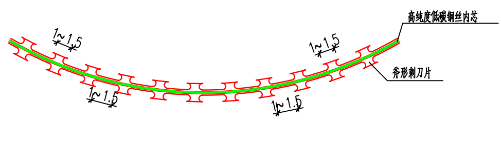
条形刺刀圈构造尺寸大样图（1：2）
